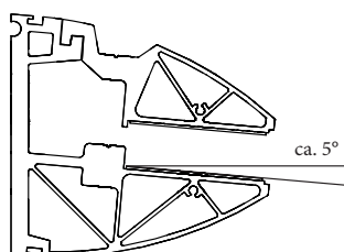
Profil DURA PLUS (Dachneigung 0°) mit Klemmprofil
