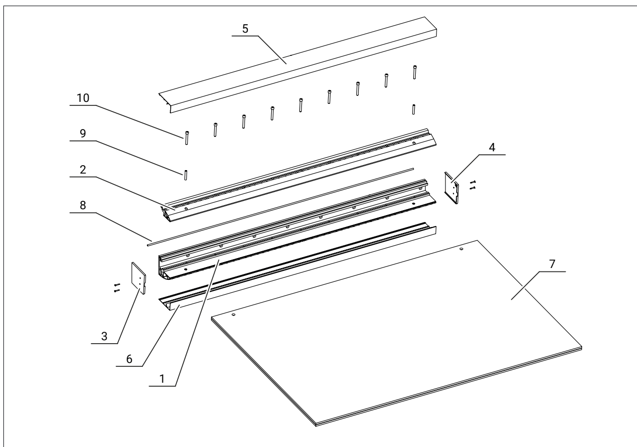
Profil DURA PLUS (Dachneigung ca. 5°) mit Klemmprofil
