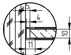
EINZELHEIT D
