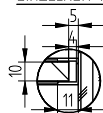
EINZELHEIT E
