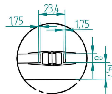
Türdichtung Griffseite
