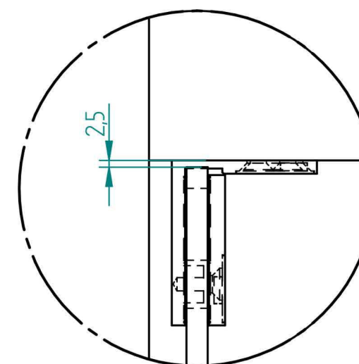
EINZELHEIT C
