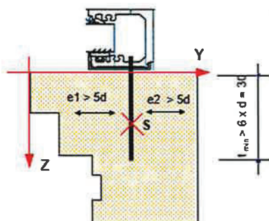
S = Schwerpunkt Schraubenbild
